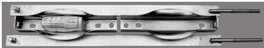
Fissaggio della cinghia sul supporto Nylstop M12
